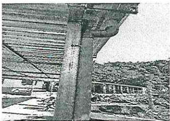
Foto 2: Sustitución de bajantes para evacuación de aguas pluviales anclada por medio de abrazaderas y tornillos
