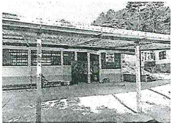
Foto1: Sustitución de cubierta de techo con lámina galvanizada, Tipo de lamina: troquelada Calibre: 26, incluye: fijaciones y sellado en traslapes.
