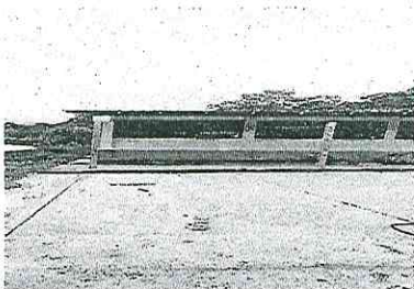
Foto 4: Reparación de losa de concreto para patios, considerando preparación de terreno, armado, nivelación y acabado rustico.
